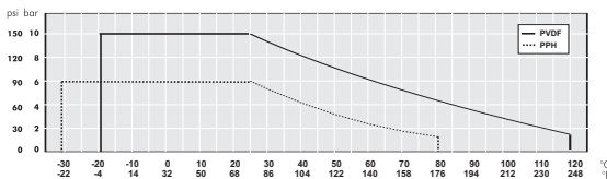
DN65 - DN80 (PPH, PVDF)
