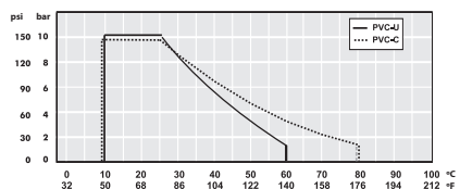
DN65 - DN80 (PVC-U, CPVC)
