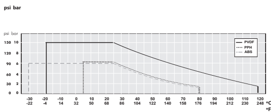
DN65 - DN80 (PPH, PVDF)
