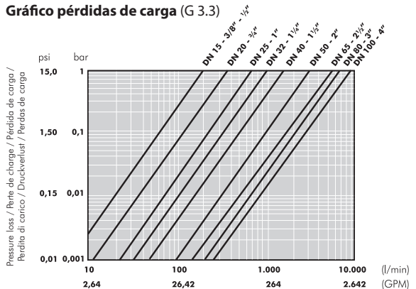
Gráfico pérdidas de carga (G 3.3)
