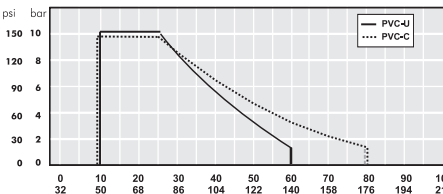
DN65 - DN100 (PVC-U, CPVC)
